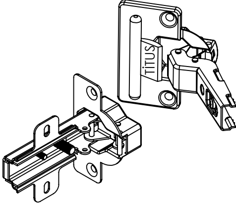
MENTEŞE (9 ADET)
